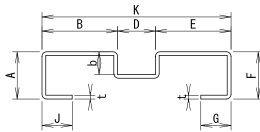
断面形状
