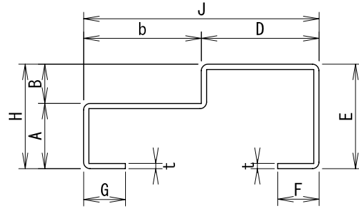
断面形状
