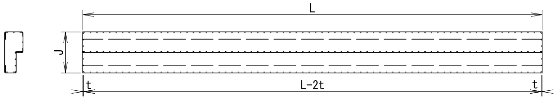
全体図(小口蓋付)
