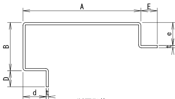
断面形状
