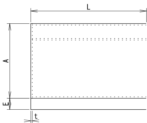
小口蓋詳細
