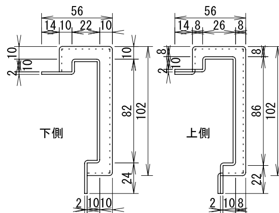
連結型小口断面寸法記入例
