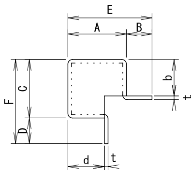
小口蓋詳細
