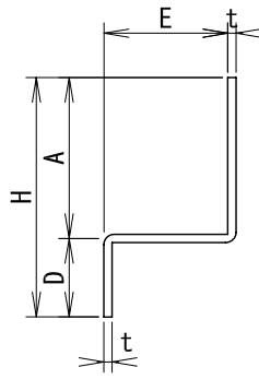
断面形状
