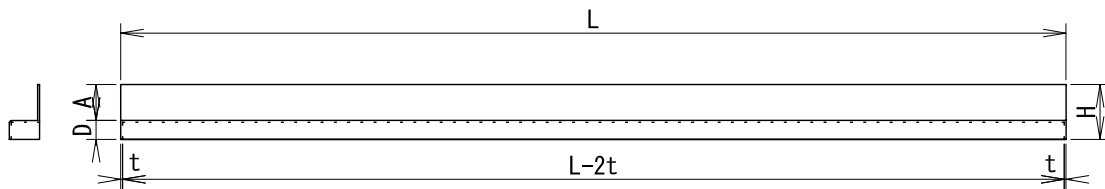
全体図(小口蓋付)
