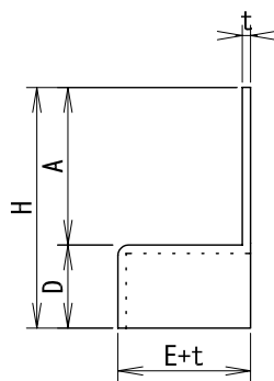
小口蓋詳細
