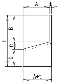
小口蓋詳細
