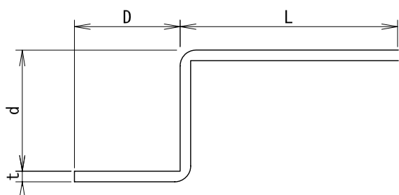
J タイプ詳細
