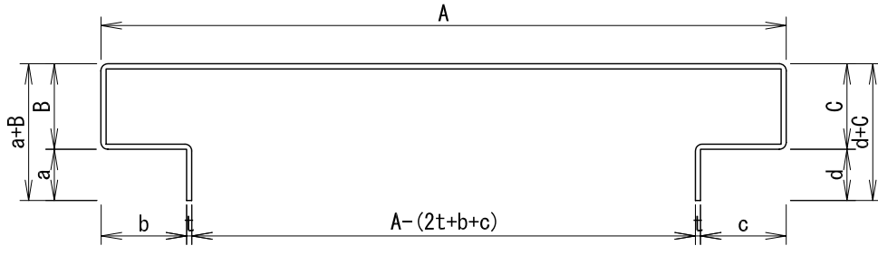
断面形状
