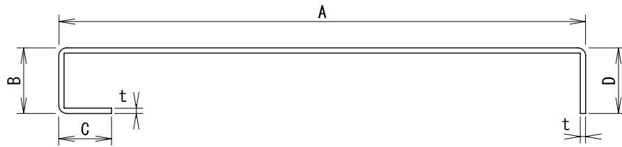
断面形状
