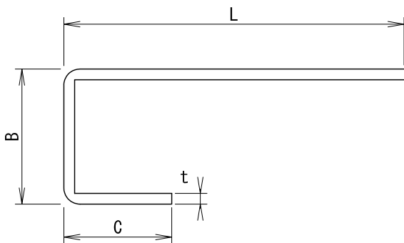
J タイプ小口蓋詳細
