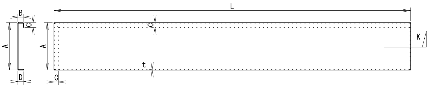
全体図
