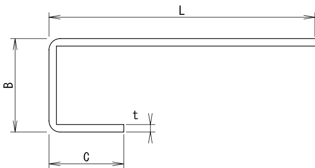
Jタイプ小口蓋付詳細図
