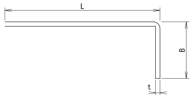
Mタイプ小口蓋付詳細図
