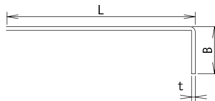
M タイプ小口蓋詳細
