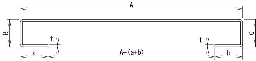
断面形状
