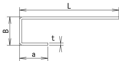
J タイプ小口蓋詳細
